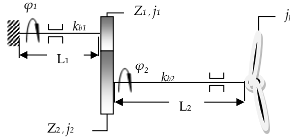
Şekil 2. Gemi sevk sistemine ilişkin matematik model
