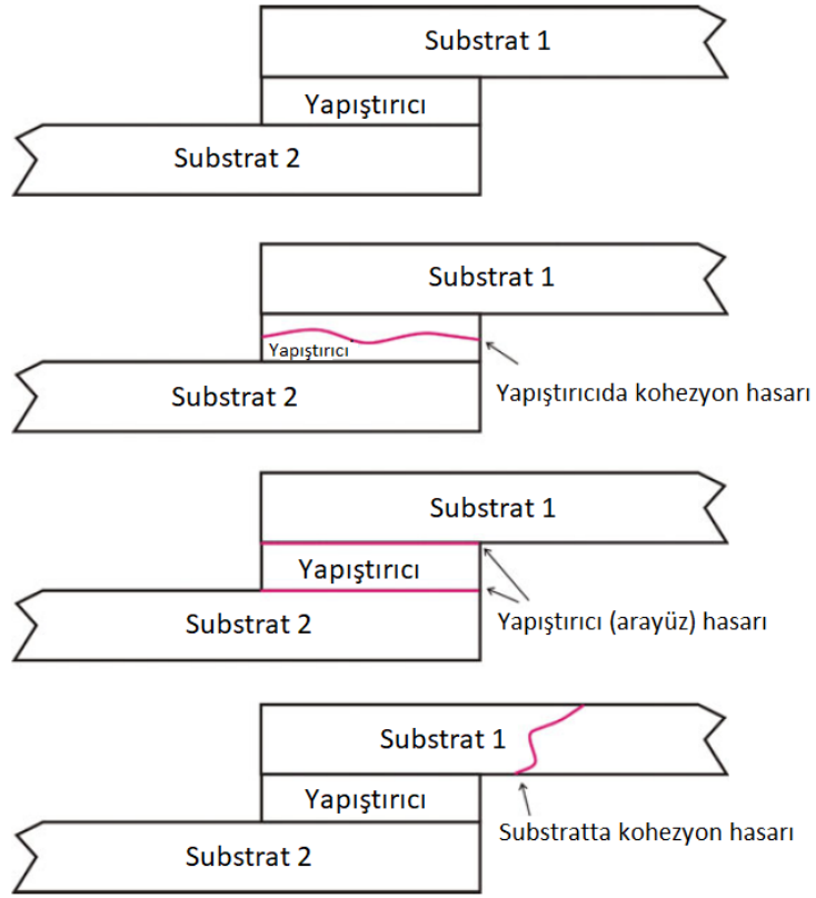
Şekil 1. 4 : Yapıştırıcı ve kohezyon hasarı gösteren yapıştırma bağlantılarından örnekler [8].
