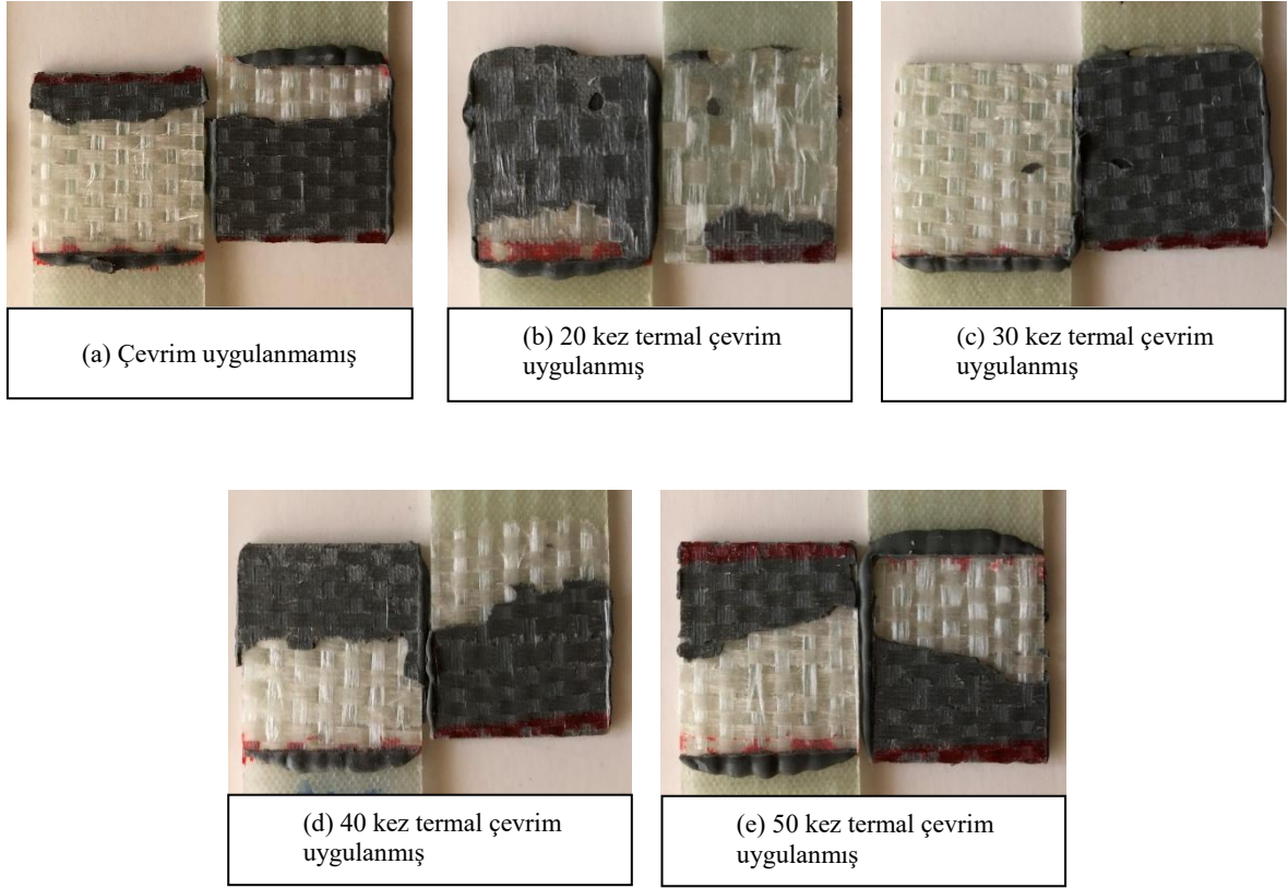
Şekil 4. 19 : Loctite 9461 ile yapıştırılmış, -10 ila 100 °C aralığında termal çevrim uygulanmış numunelere ait tipik kırılma yüzeyleri.
