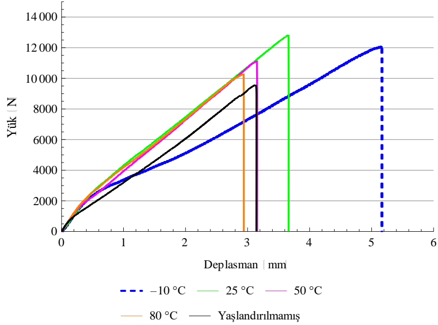
Şekil 4. 43 : DP 460 ile yapıştırılmış, 168 saat yaşlandırılmış numunelere ait Yük - Deplasman eğrileri.
