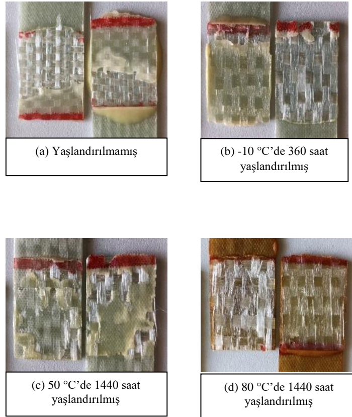
Şekil 4. 50 : DP 460 ile yapıştırılan numunelere ait kırılma yüzeyleri.
