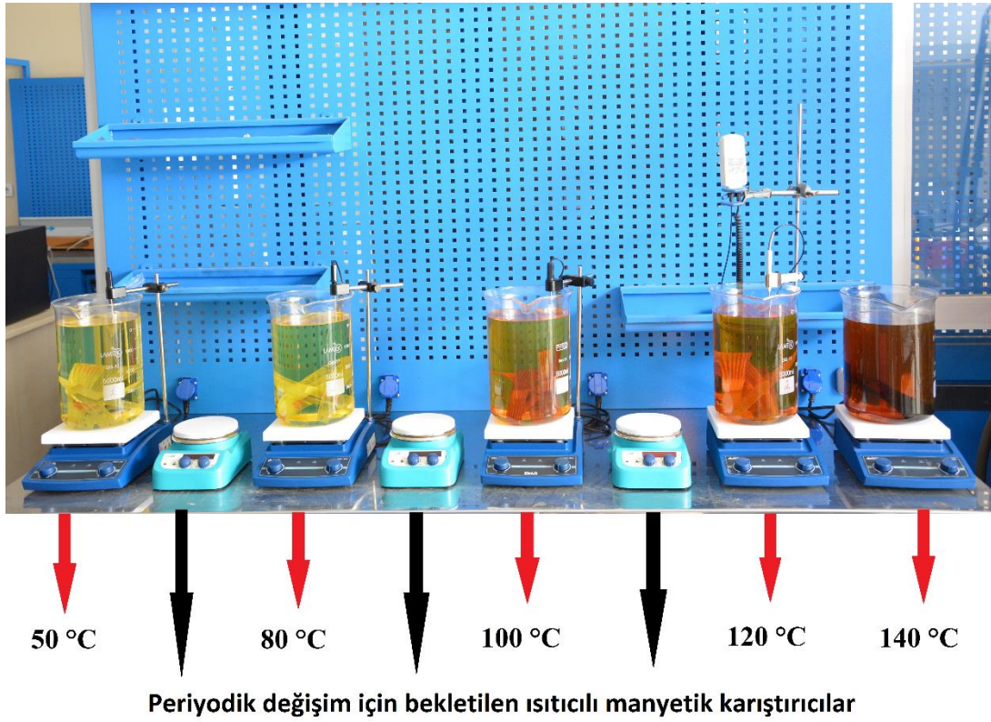
Şekil 3. 21 : Termal-yağ yaşlandırma deney düzeneği.
