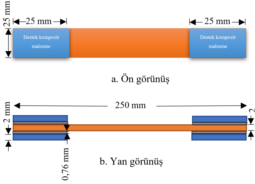
Şekil 3. 5 : ASTM D3039'a göre hazırlanmış olan numunenin şematik görünüşü.
