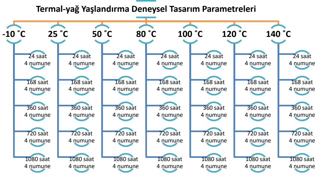
Şekil 3. 23 : Termal-yağ yaşlandırma deneysel tasarım parametreleri şematik gösterimi.
