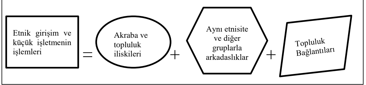
Şekil 2: Sade Doğrusal Model “Simple Linear Model”
