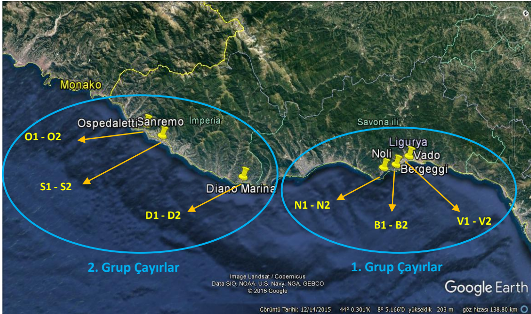
Şekil 2.1.2. Ligurya Denizi'nde çayrların dağılımı.
