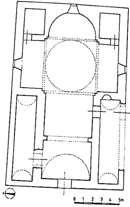
Şekil 9: Artvin Dolishane (Hamamlı) Kilisesi Plan (O. Aytekin, 1999, s. 59)
