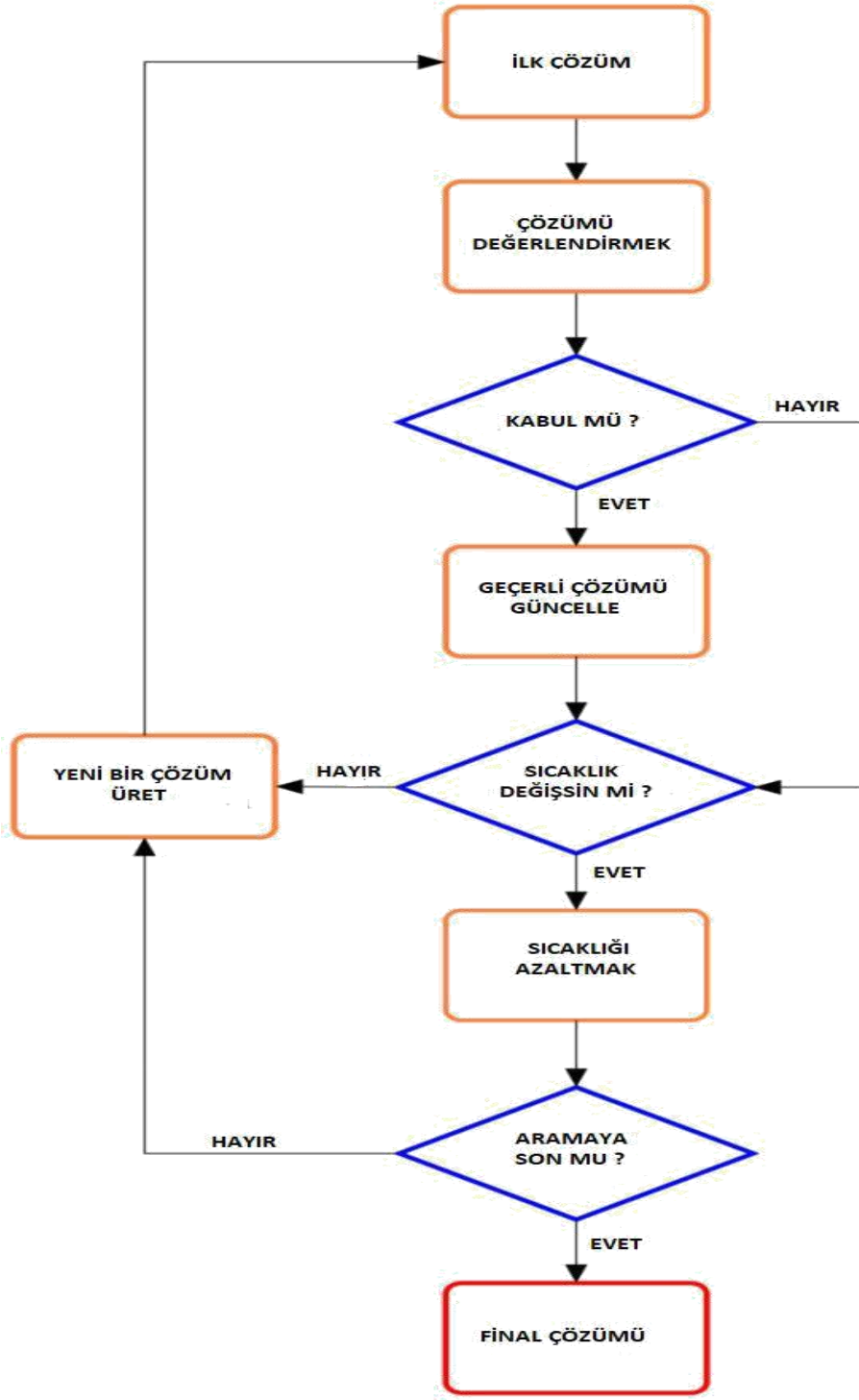
Şekil 5.3 : Simulated Annealing akış şeması [75]
