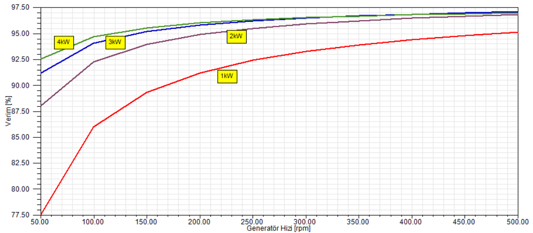
Şekil 7.8: Farklı Güçlerde Hıza Bağlı Verim
