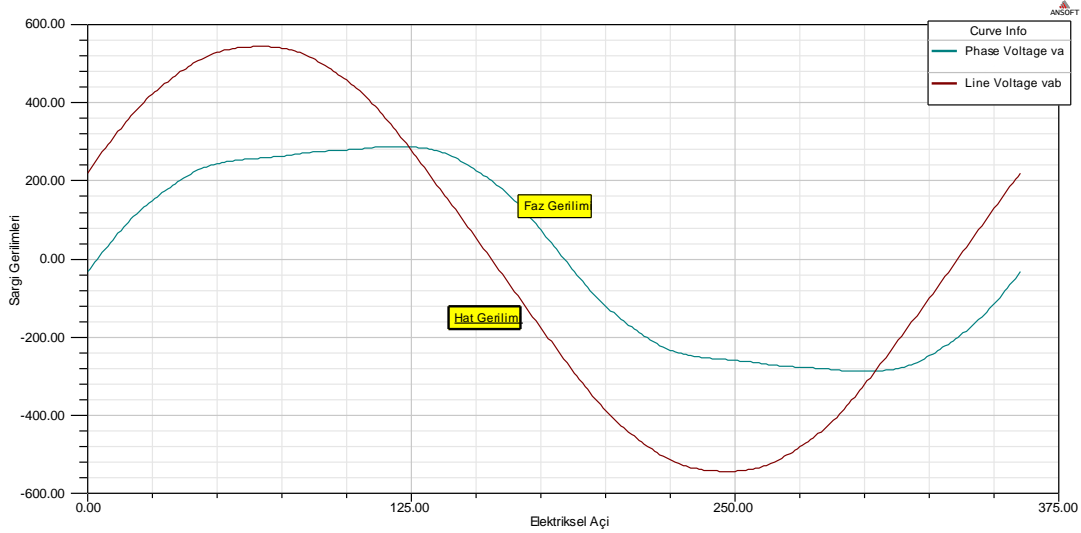
Şekil 7.6: Elektriksel Açığa Bağlı Sargı Gerilimleri
