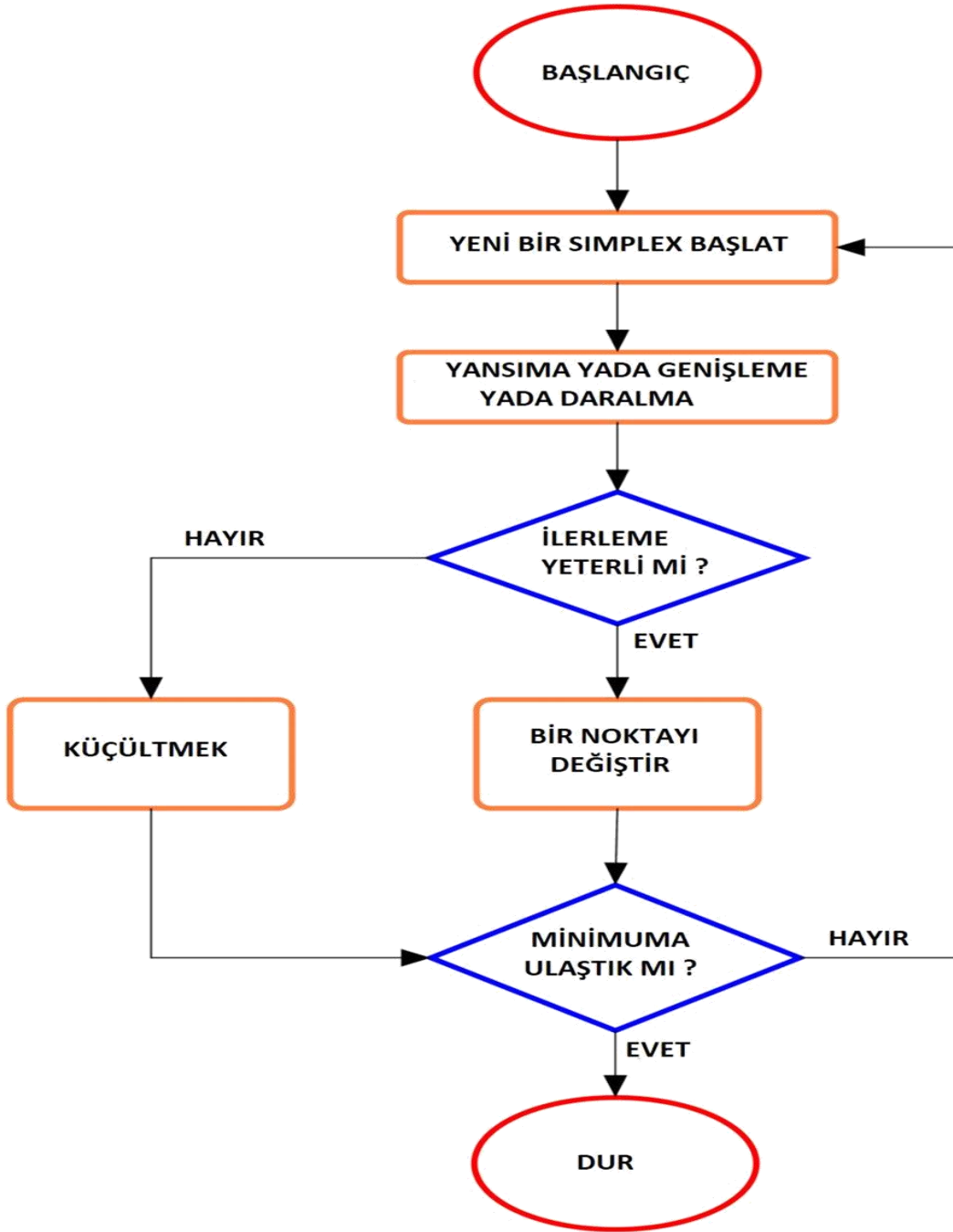
Şekil 5.1 : Nelder-Mead akış şeması [72]
