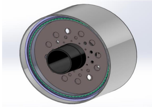
Şekil 2.3: In-runner bir SMSG'nin 3D tasarımı
