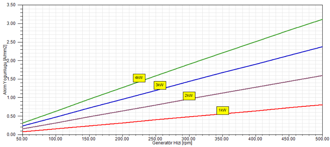
Şekil 7.9: Farklı Güçlerde Hıza Bağlı Akım Yoğunluğu
