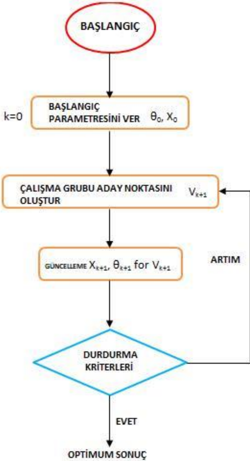
Şekil 5.2 : Random Search akış şeması [73]
